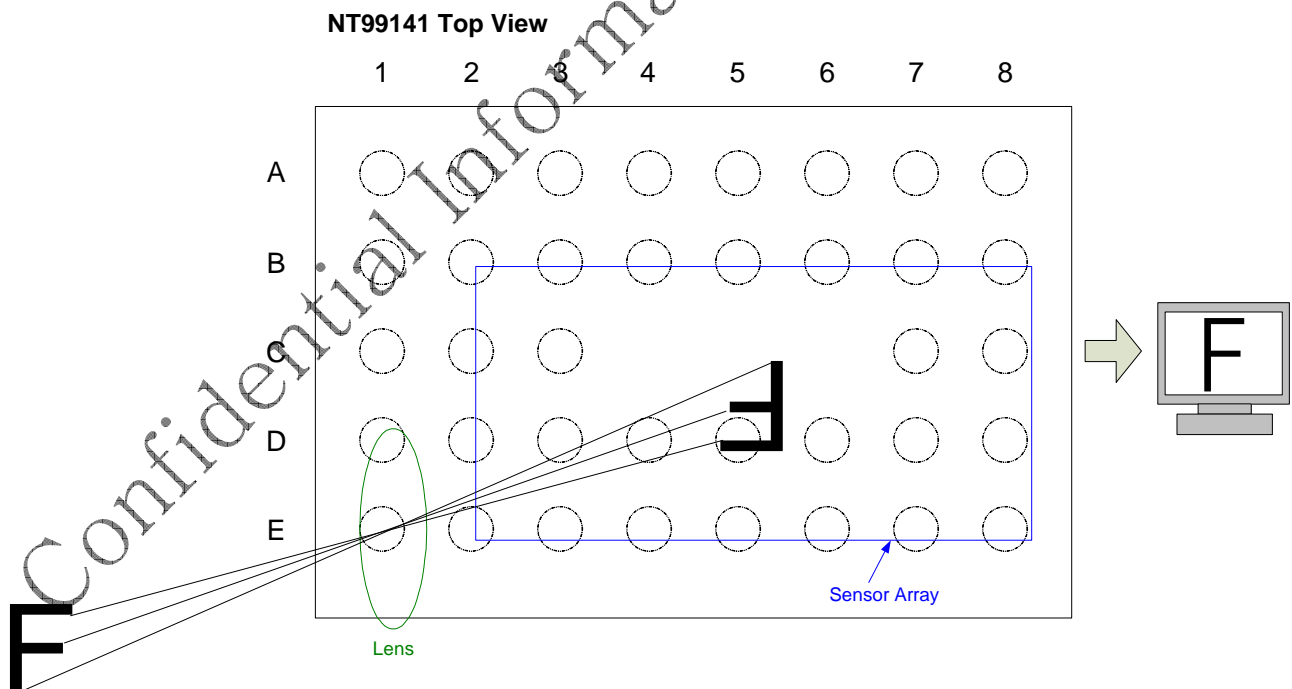
Fig. 12 Default Readout Order
